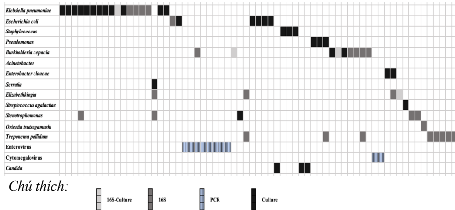
Hình 4.1. So sánh kết quả chẩn đoán tác nhân gây bệnh giữa các phương pháp
