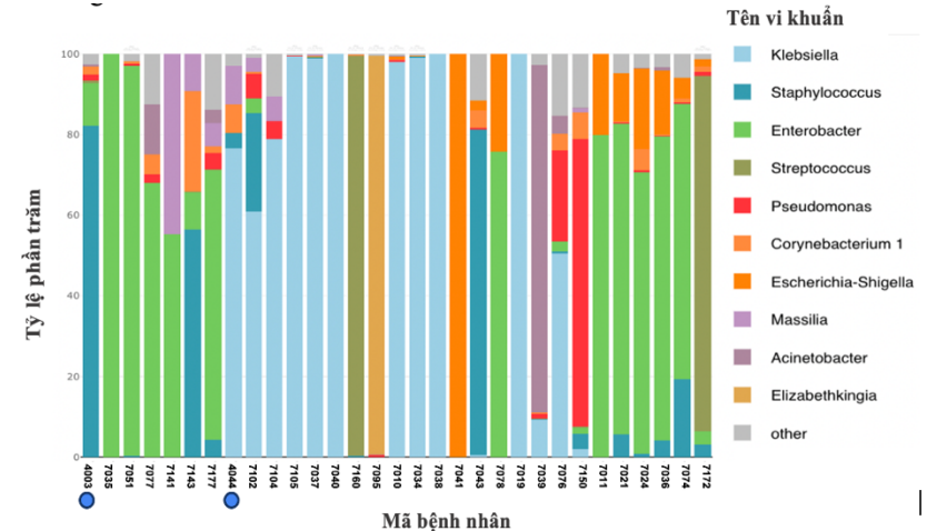
Hình 3.1. Phân bố tác nhân vi khuẩn nghi ngờ gây bệnh trong mẫu dịch não tủy
